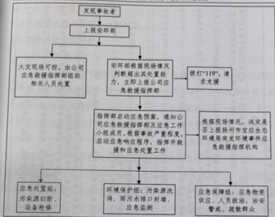
图2 火灾引发二次污染事件应急处置程序图
